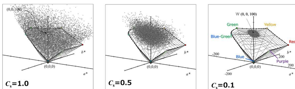
図5.5 カラースペックルの計算結果のCIE Lab空間表示
