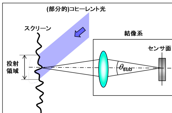
図2.2 結像系スペckル
