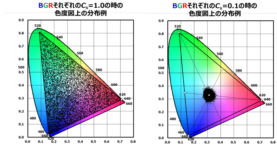
図2.6 カラースペックルの色空間(CIE 1931)での分布例
