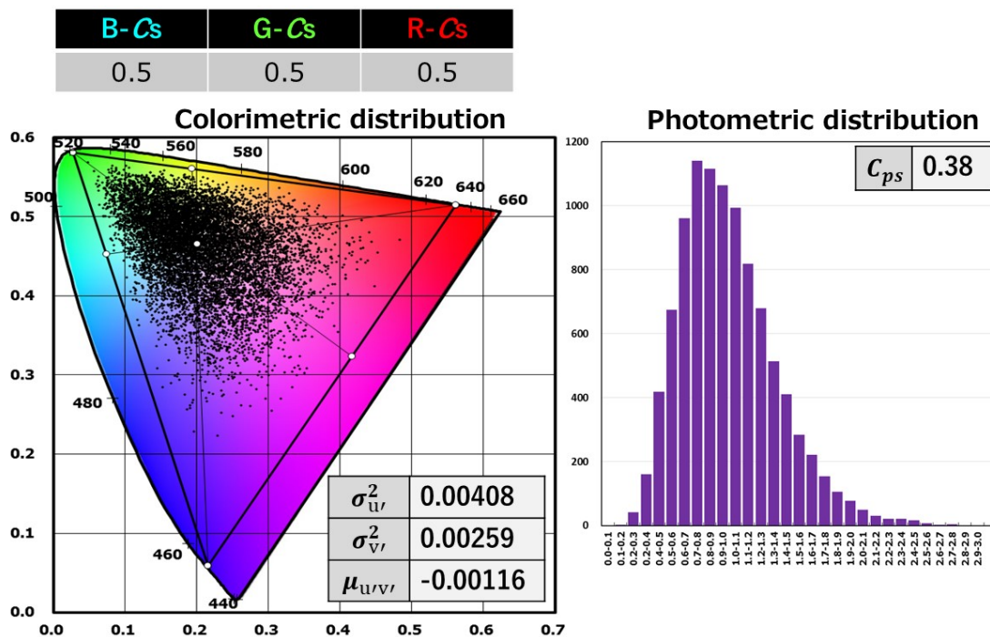
図5.3 カラースペックルの計算結果の例 (R、G、Bの C_s =0.5)
