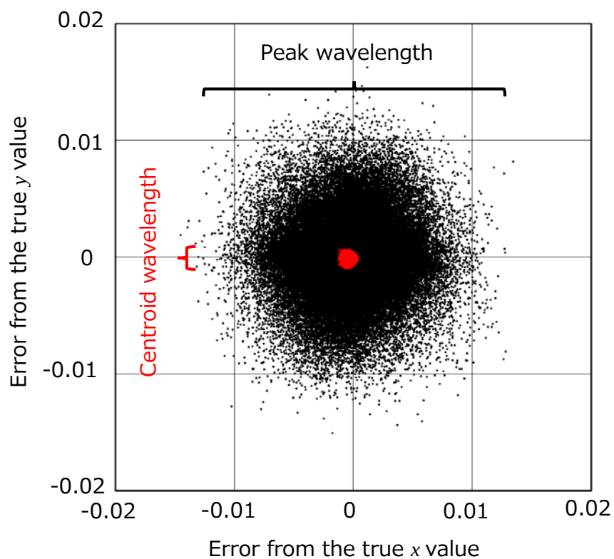
図4.5 重心波長とピーク波長を使った場合の色度誤差比較
