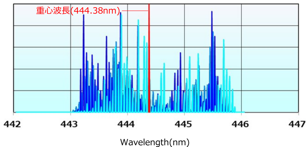
図4.4 複数のマルチ縦モードの分布
