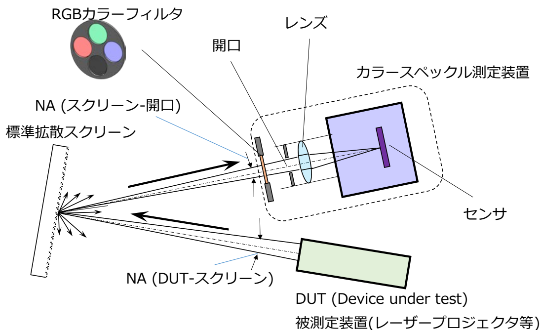
図5.6 カラースペックルの測定装置の構成
