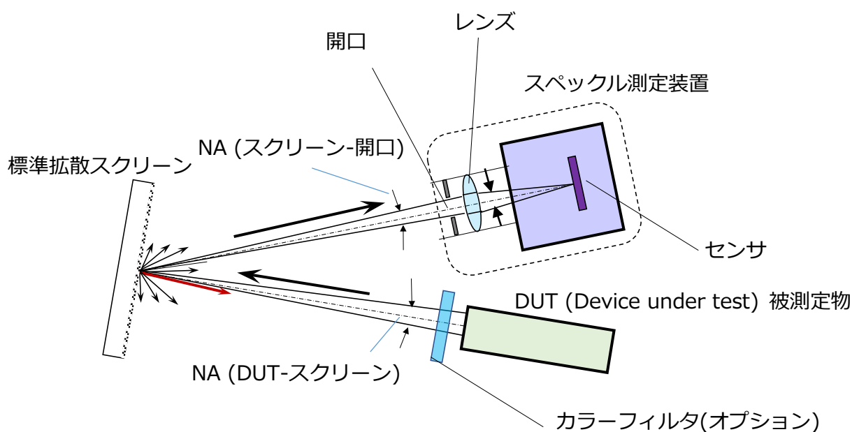
図3.2 単色speckルの測定装置の構成
