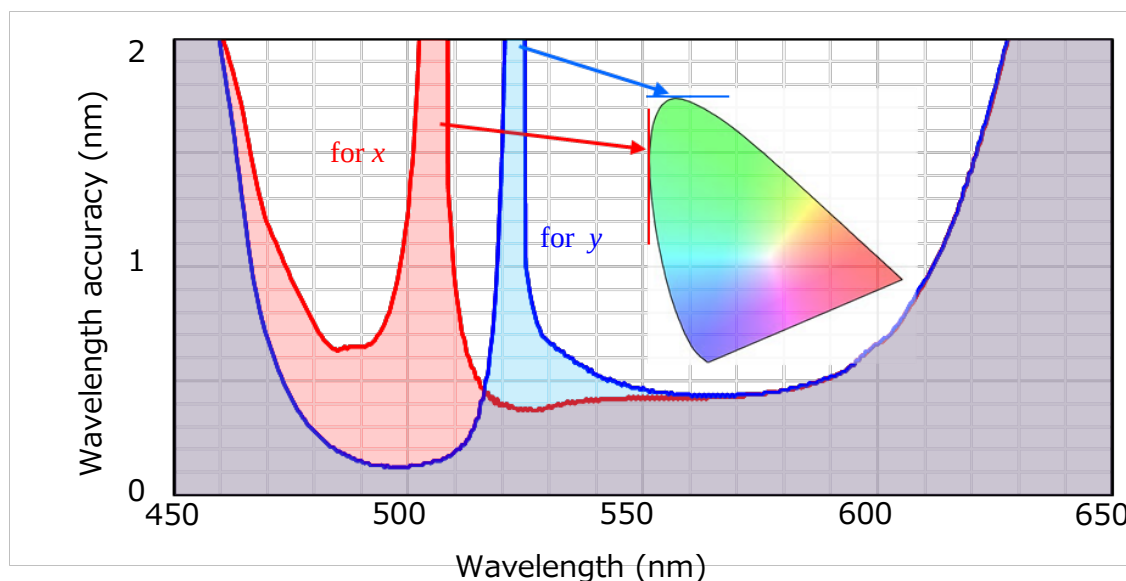
図4.3 \Delta x, \Delta y < 0.003 の色度精度が得られる波長精度の波長についてのプロット
