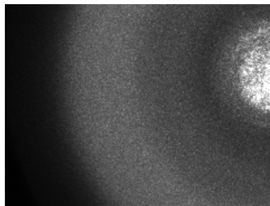
図2.3 ファイバースペックルパターン(ファイバー: MMF)が乗ったスクリーンスペックルの観測例
