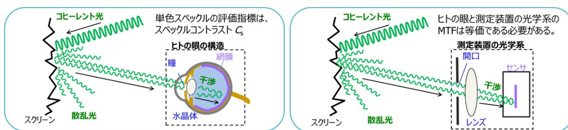
図3.1 人間の眼の結像系と測定装置の結像系
