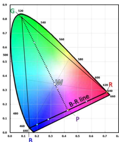
図 A.1 パワー比を求める方法を説明する色度図
