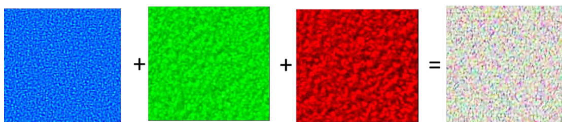
図 5.1 RGB 単色スペckルの加法混色(カラースペckル)
