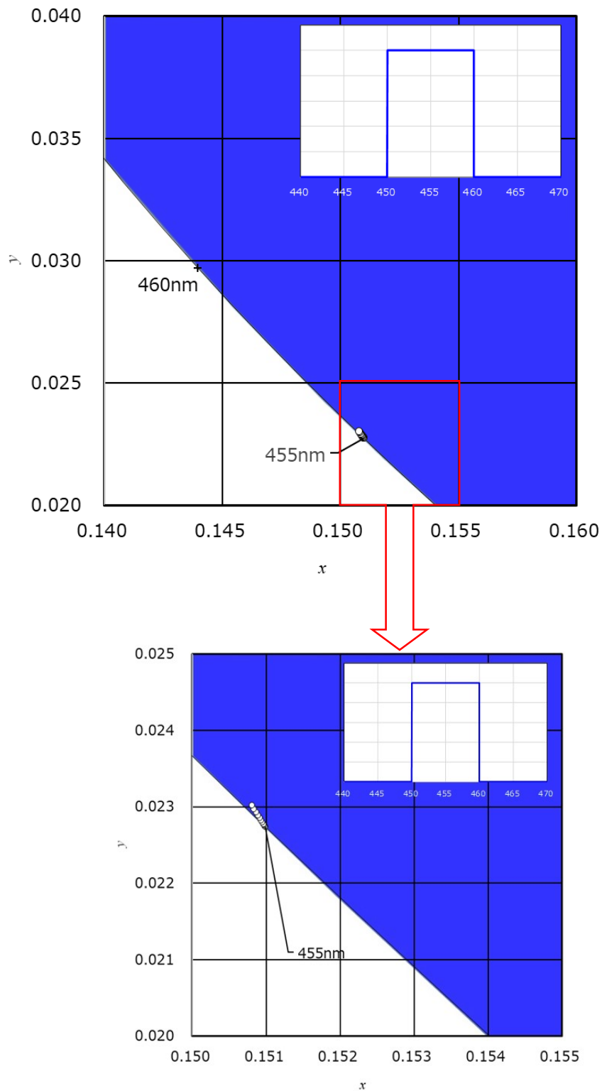
図4.2 矩形型スペクトルの半値幅と色度の関係
