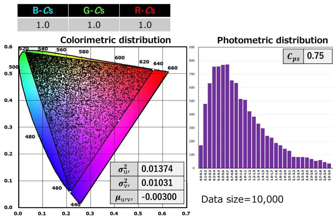
図5.2 カラースペックルの計算結果の例 (R、G、Bの C_s =1.0)
