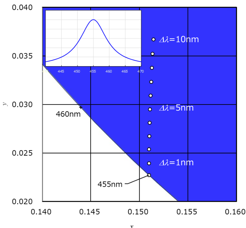
図4.1 ローレンツ型線スペクトルの半値幅と色度の関係
