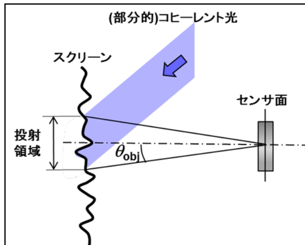
図2.1 非結像系スペckル
