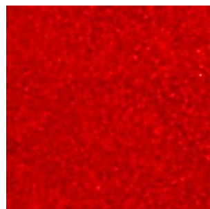
図2.4 単色スペックルパターン
